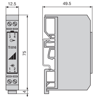
Fig. 10. SINEAX TI 816 on top-hat rail EN 50 022 – 35×7.5.
