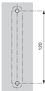
Fig. 7. Plan de perçage.
