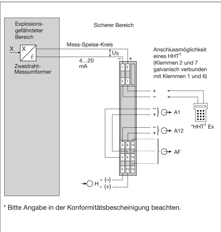
Bild 9. SINEAX Typ 811-1..0 .... , Mess-Speise-Kreis eigensicher, Speisespannung U_s 16,9 V DC, nicht FSK-durchgängig.
