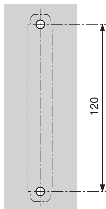
Bild 7. Bohrplan.
