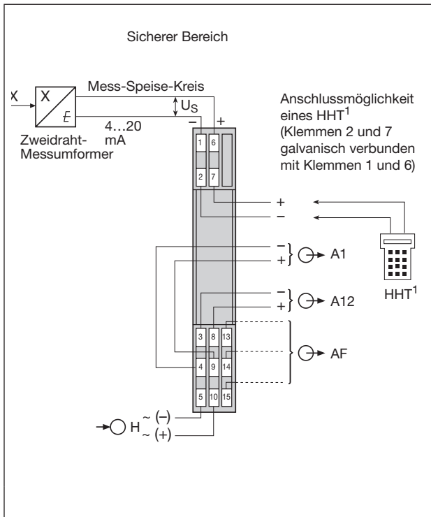
Bild 8. SINEAX Typ 811-1..0 .... , Mess-Speise-Kreis und Ausgang nicht eigensicher, Speisespannung U_s 24 V DC, nicht FSK-durchgängig.
