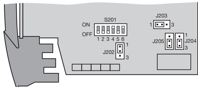
Bild 14. Anordnung des Dip-Schalters S 201 und der Jumper J 202 bis J 205.
