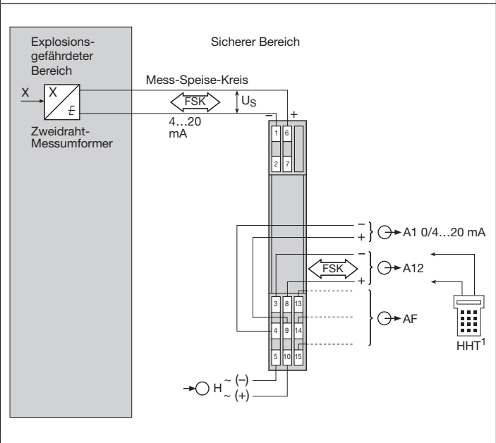
Bild 11. SINEAX Typ 811-1..1 .... , Mess-Speise-Kreis eigensicher, Speisespannung U_s 16,4 V DC, FSK-durchgängig. Hand-Held-Terminal an Feldausgang A12 angeschlossen.
