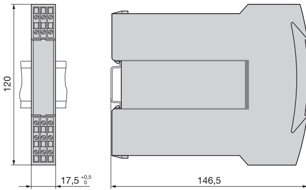
Fig. 16. SINEAX B 811 en boîtier S17 encliqueté sur rail symétrique (35 x 15 mm ou 35 x 7,5 mm, selon EN 50 022).
