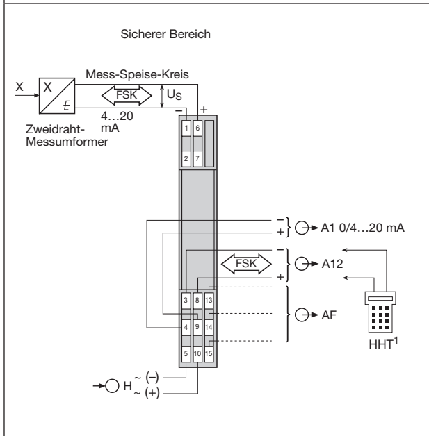
Bild 10. SINEAX Typ 811-1..1 .... , Mess-Speise-Kreis und Ausgang nicht eigensicher, Speisespannung U_s 24 V DC, FSK-durchgängig. Hand-Held-Terminal an Feldausgang A12 angeschlossen.
