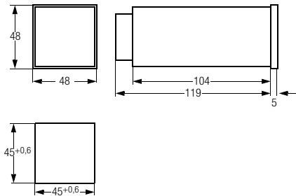
Figure 1, Dimensions du boîtier et découpe du panneau de commande
