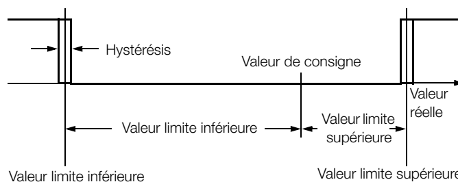
Fig. 2 Représentation schématique de la surveillance valeur limites relatives
