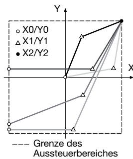
Bild 9. Beispiele für Einstellmöglichkeiten bei geknickter Kennlinie.
